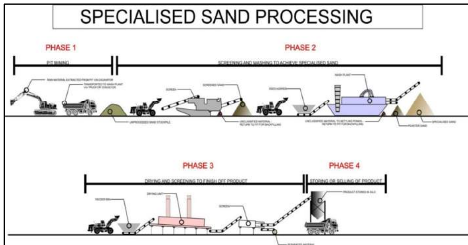
Figuur 2: Gespesialiseerde sandverwerking.
