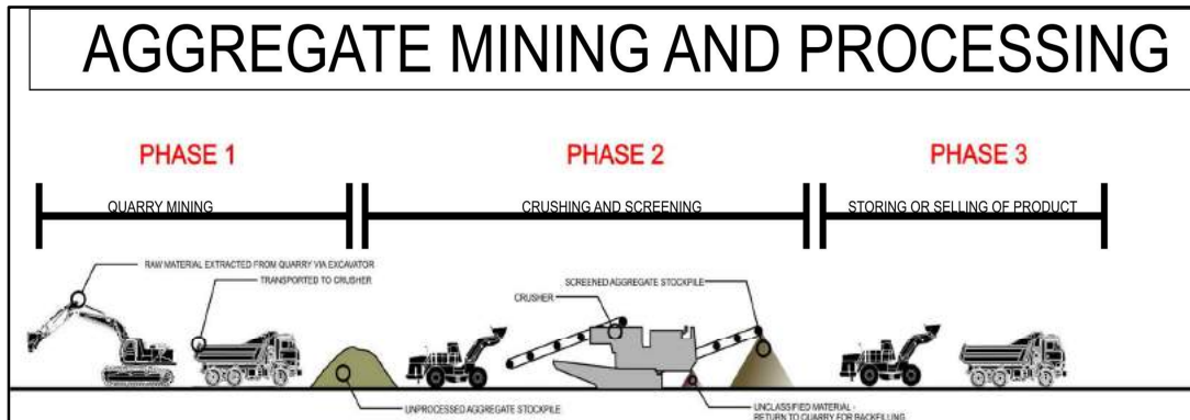
Figuur 3: Aggregaat-ontginning en -verwerking.
