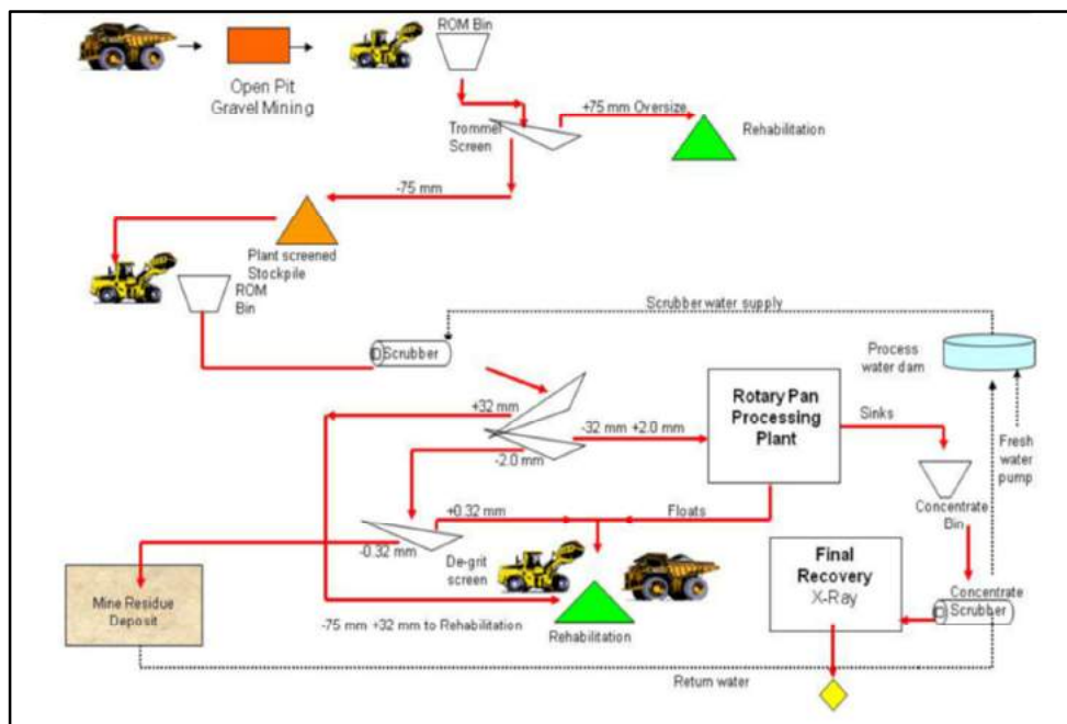
Figuur 4: Diamantontginningsmetode.
